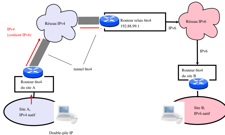
FIG. 7 – Scénario 6to4
