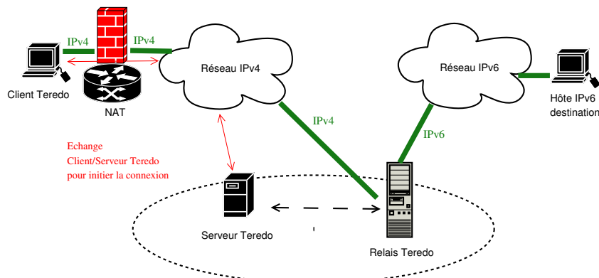
FIG. 8 – Exemple Teredo
