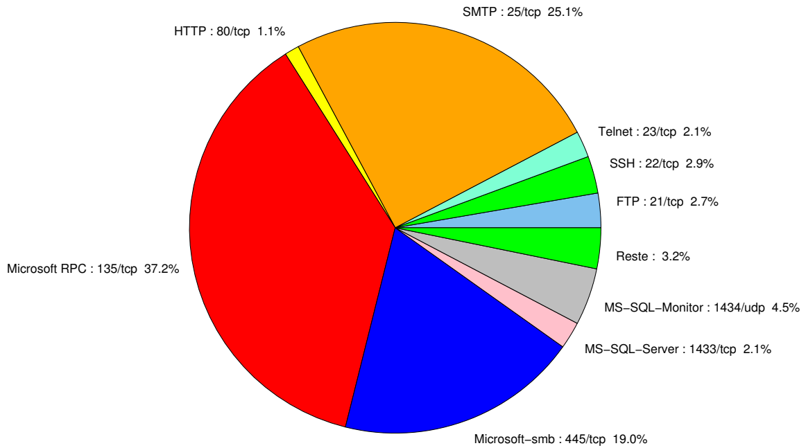
FIG. 1: Répartition relative des ports pour la semaine du 10 au 17 septembre 2009
